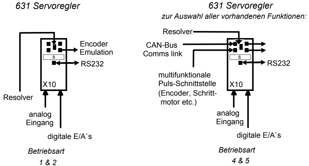
Abbildung 4-1 Anschlussbeispiele
