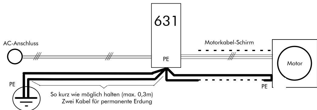
Abbildung 12-1 EMV und Sicherheitserdung
