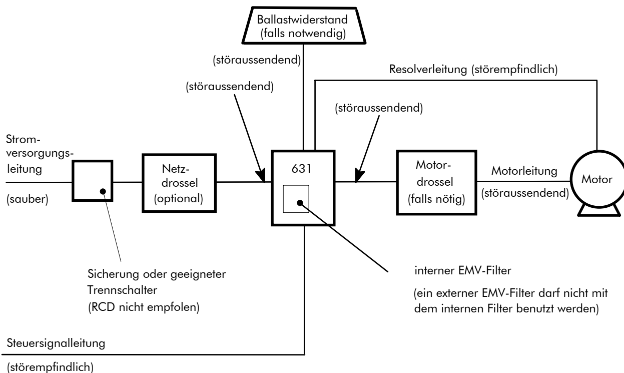
Abbildung 3-2 Verkabelungsanforderungen
