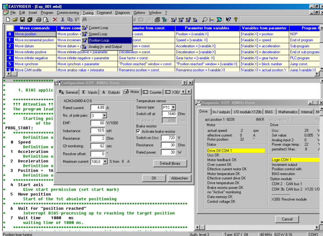
Abbildung 6-1 EASYRIDER Hauptbildschirm
